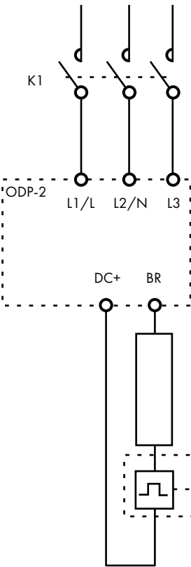
带内部超温开关的热过载/制动电阻器
