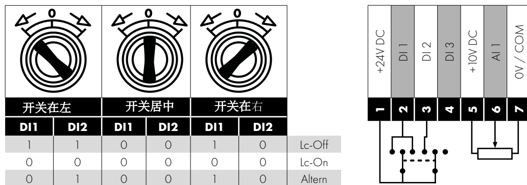
开关和电位器
